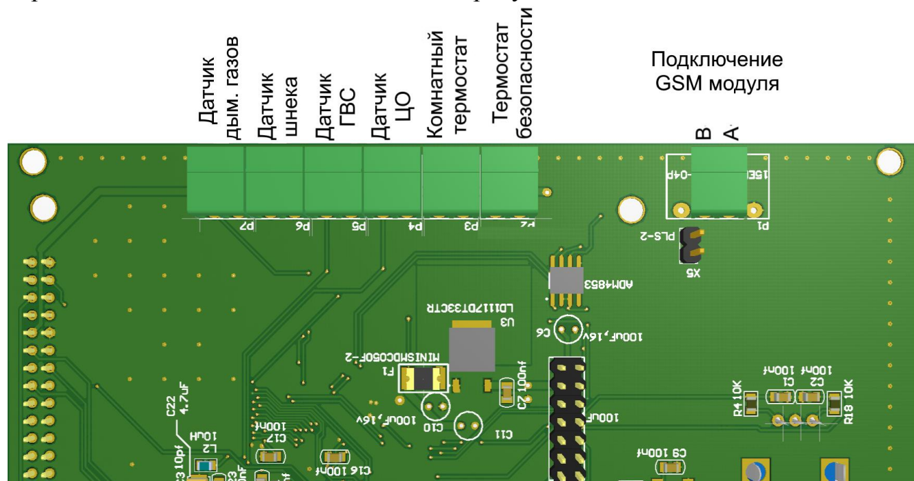
Рис. 22 – Схема подключения датчиков, комнатного термостата, термостата безопасности и GSM модуля
