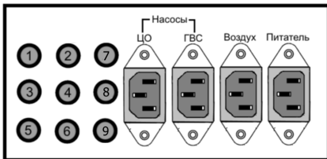
Рис. 2 – Задняя панель контроллера.
