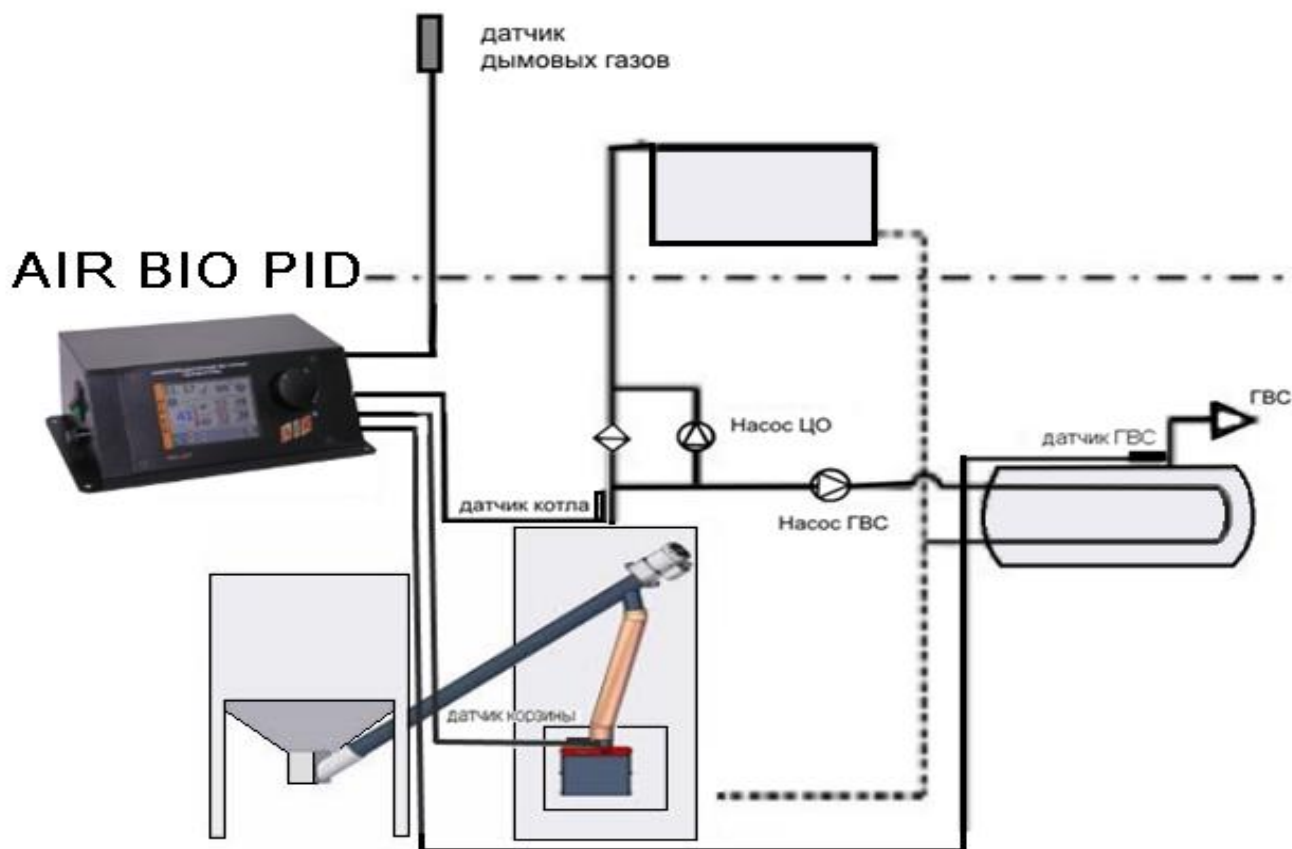
Рис.1 - Схема подключения AIR BIO.
