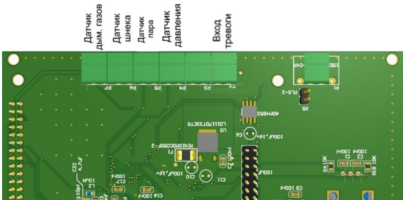
Рис. 22 – Схема подключения датчиков, комнатного термостата, термостата безопасности и GSM модуля
